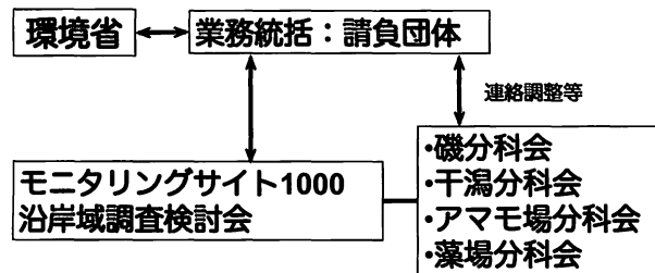
図1 環境省モニタリングサイト 1000 沿岸域調査の実施体制。2007 年から 2011 年の請負団体は、特定非営利活動法人日本国際湿地保全連合（WIIJ）。
