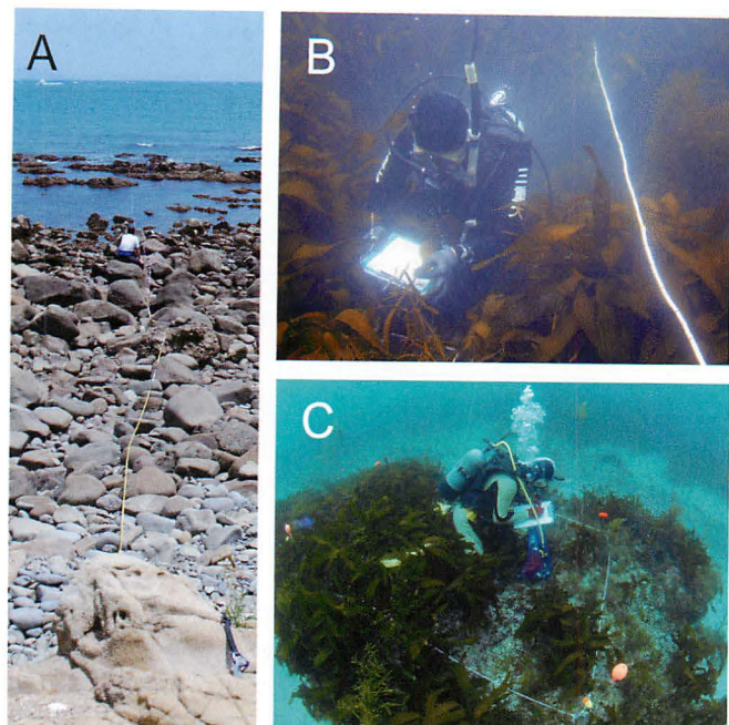
図4 環境省モニタリングサイト 1000 沿岸域調査における藻場調査風景。A 調査測線の設置（兵庫県洲本市由良）、B 測線上での出現種の被度調査（同左）、C 永久方形枠での出現種の被度調査（兵庫県豊岡市竹野）。
