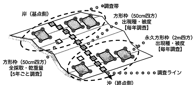
図3 環境省モニタリングサイト 1000 沿岸域調査における藻場調査の模式図。調査はライントランセクト調査と永久方形枠の被度調査、生物量の定量調査で構成される。
