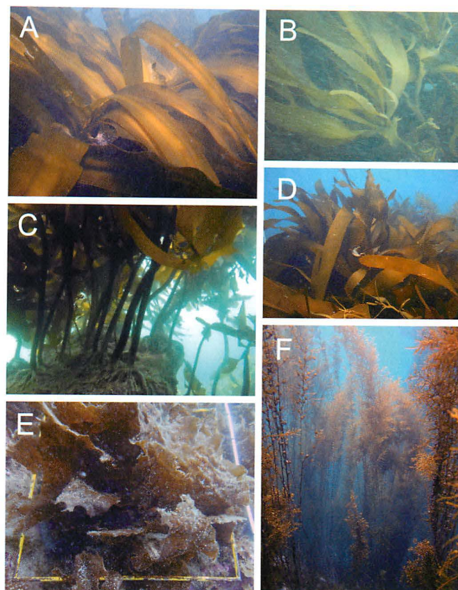
図5 環境省モニタリングサイト 1000 沿岸域調査で見られた各調査サイトの藻場景観。A 北海道室蘭市のコンブ群落、B 宮城県南三陸町志津川のアラメ群落、C 静岡県下田市のカジメ群落、D 兵庫県洲本市由良のカジメ群落、E 鹿児島県長島町のアントクメ群落、F 兵庫県豊岡市竹野のヤツマタモク群落（周辺にはクロメも混生する）。
